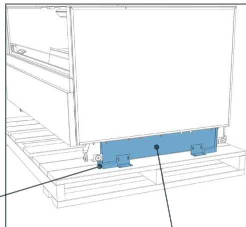
Support d'expédition
